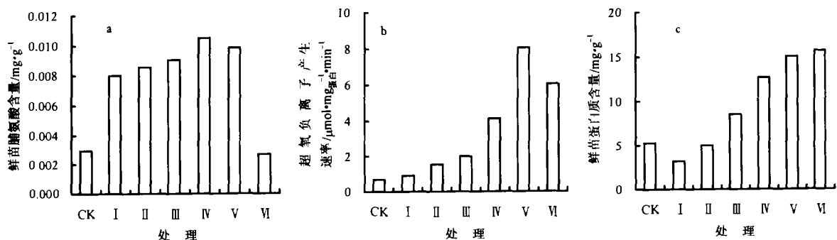
图1 Cr^{3+} 胁迫对木麻黄幼苗脯氨酸、超氧负离子和蛋白质含量的影响
