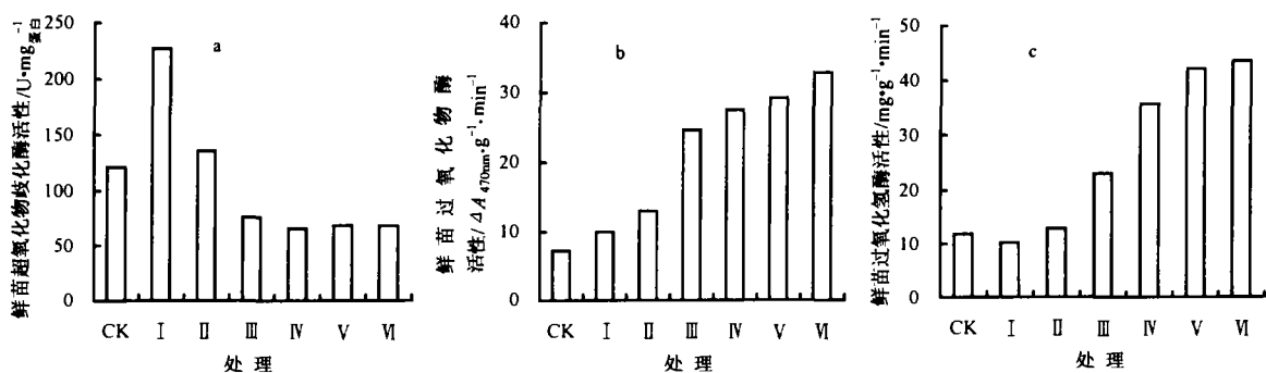
图 2 \text{Cr}^{3+} 胁迫对木麻黄幼苗 SOD、POD 及 CAT 活性的影响
